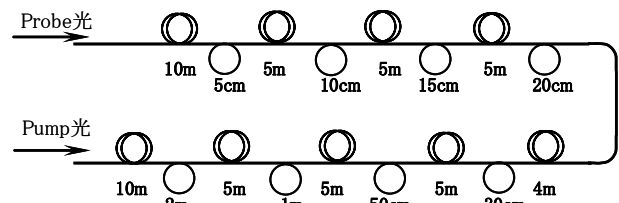
図6 被測定ファイバの構成
